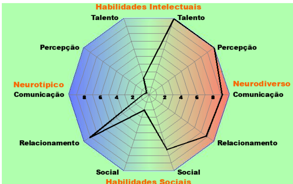
Imagen 2. Aspie Quiz
